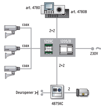
Variant met extra camera's voor eengezinswoningen
