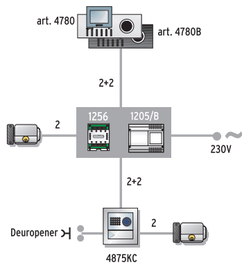
Variant met extra elektrisch slot voor eengezinswoningen
