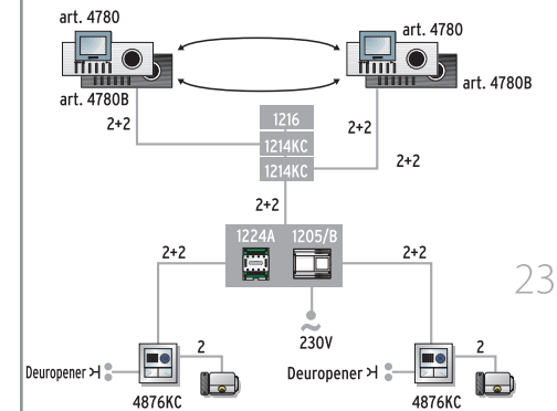
Variant met tweede entreepaneel voor de Divakit voor tweegezinswoningen
