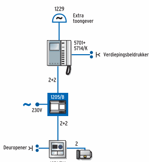
Variant met aansluiting van een verdiepingsebelddrukker en extra toongever voor Bravokit voor een- en tweegezinswoningen
