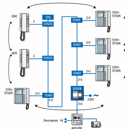
Variant met twee monitoren of twee extra audiotoeestellen voor Bravokit voor tweegezinswoningen
