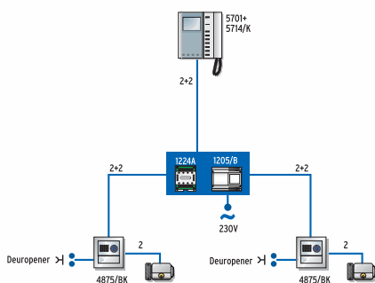
Variant met tweede entreepaneel voor de Bravokit voor eengezinswoningen
