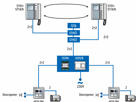
Variant met tweede entreepaneel voor de Bravokit voor tweegezinswoningen
