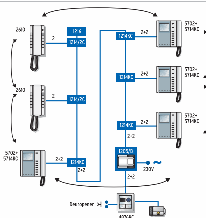
Variant met twee monitoren of twee extra audiotostellen voor Bravokit voor tweegezinswoningen
