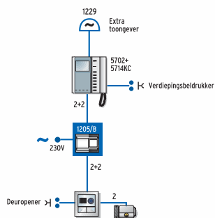
Variant met aansluiting van een verdiepingbeldrukker en extra toongever voor Bravokit voor een- en tweegezinswoningen
