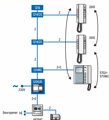
Variant met twee extra audiotostellen voor de Bravokit voor eengezinswoningen met intercomfunctie
