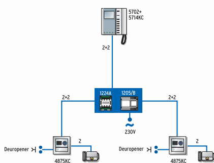
Variant met tweede entreepaneel voor de Bravokit voor eengezinswoningen
