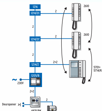
Variant met twee extra audiotoeestellen voor de Bravokit voor eengezinswoningen met intercomfunctie
