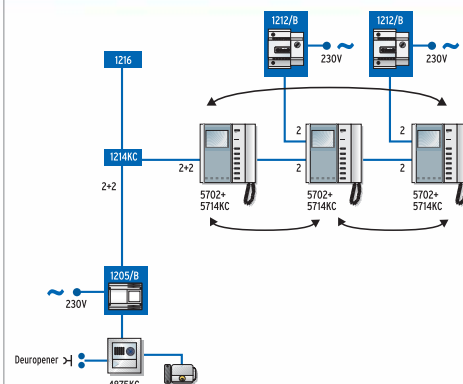
Variant met twee extra monitoren voor de Bravokit voor eengezinswoningen
