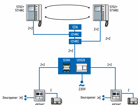
Variant met tweede entreepaneel voor de Bravokit voor tweegezinswoningen
