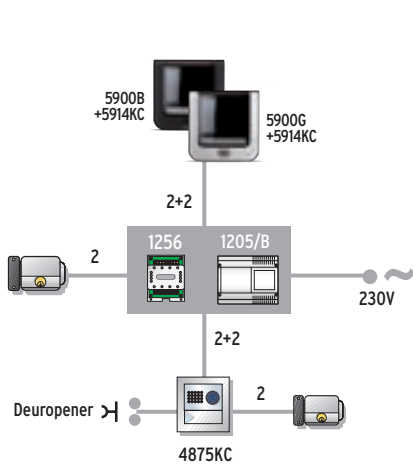
Variante met extra slot voor eengezinswoningen
