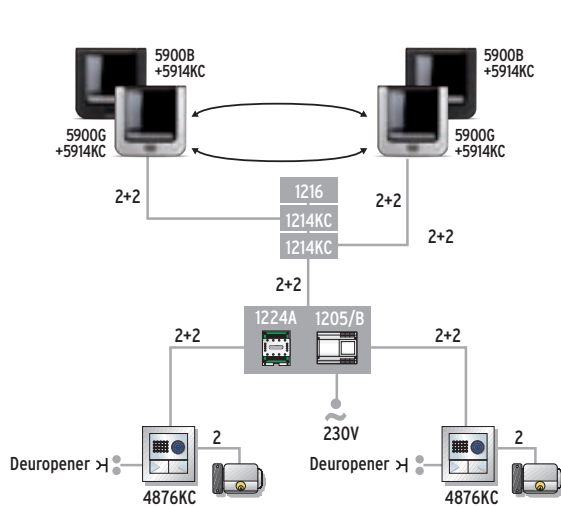
Variante met tweede entreepaneel voor tweegezinswoningen
