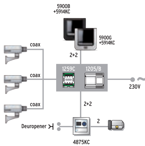
Variante met extra camera's voor eengezinswoningen
