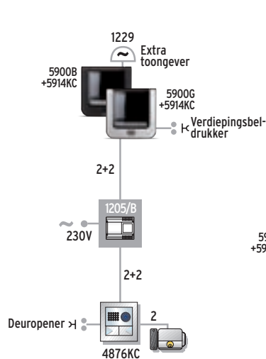
Variante met aansluiting voor verdiepingbel-drukker en extra toongever voor een- en tweegezinswoningen
