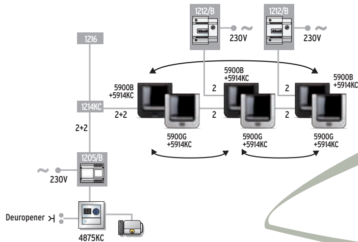
Variante met twee extra monitoren voor eengezinswoningen
