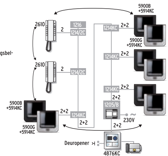
Variante met twee monitoren of twee extra audio toestellen voor tweegezinssets
